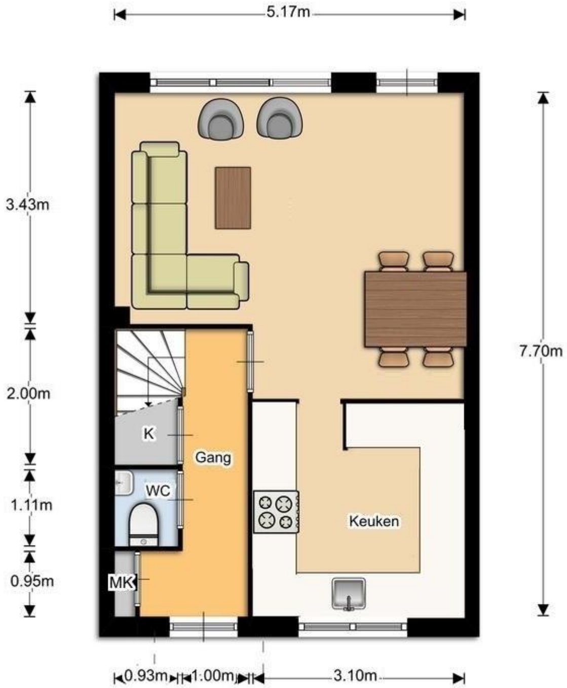
Begane Grond
